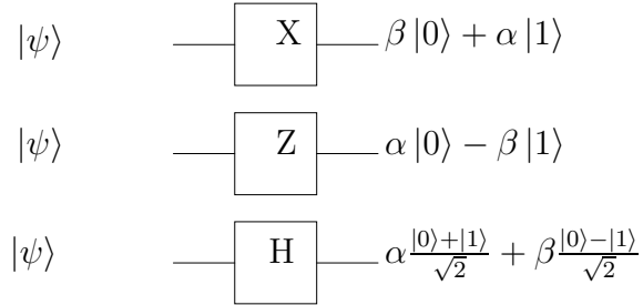
Figure 6: Le porte X , Z e H
