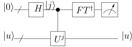
Figure 27: Circuito schematico per l'algoritmo di stima delle fasi
