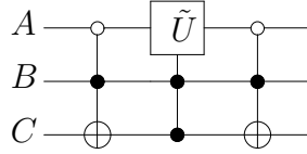
Figure 25: Circuito che implementa la matrice a due livelli U dell'esempio 12.9
